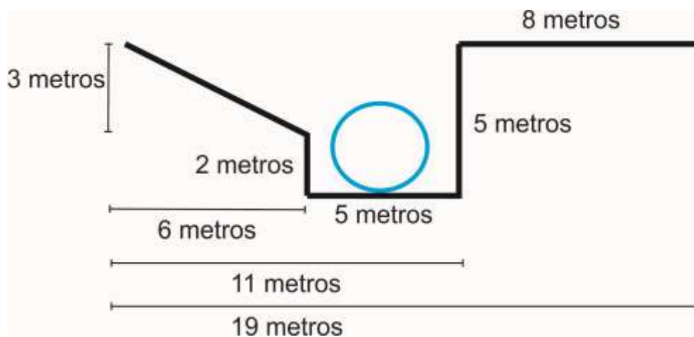
Figura 5. Esquema zanja.
